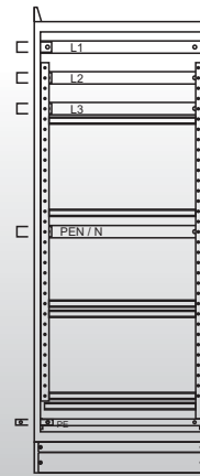
Anschlussfeld 850 mm breit
