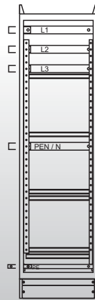
Anschlussfeld 600 mm breit
