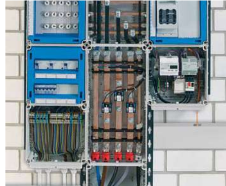
Messung mit Wandlergehäuse und Stromwandlern
