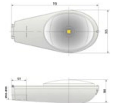
Abmessungen
