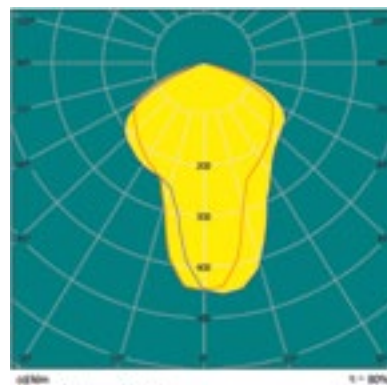
Lichtverteilung
