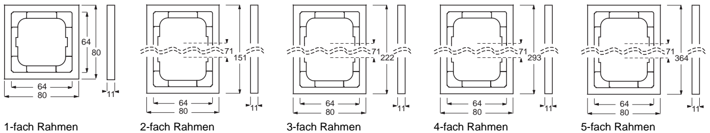
1-fach Rahmen
